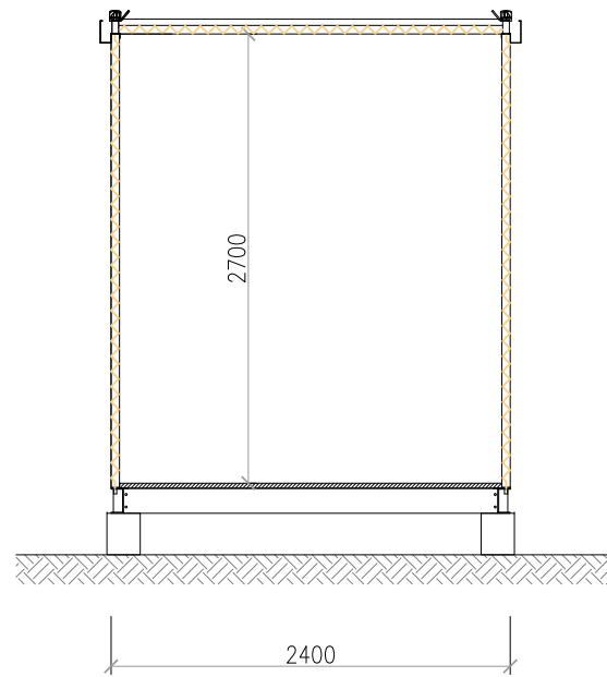
Sezione tipica
